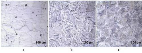
Şekil 3: Sinterlenmiş (a): saf Ti, (b): Ti-16Nb, c)Ti-26Nb alaşımlarının optik mikroyapı görüntüleri.
