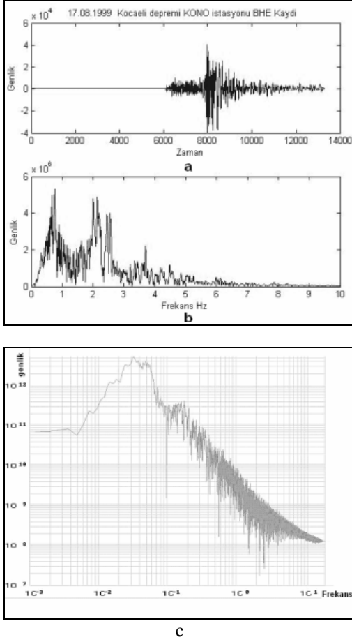
Şekil 12. a) 17.08.1999 tarihinde meydana gelen büyüklüğü M_w : 7.4 olan depremin doğu bileşen kaydı, b) Bu kayda uygulanmış Fourier dönüşümü ve c) Aynı kayda uygulanmış Fourier dönüşümü logaritmik eksenlerdeki görünümü.
