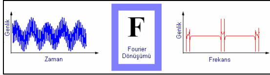
Şekil 2. Fourier dönüşümü.
