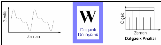
Şekil 3. Dalgacık dönüşümü.
