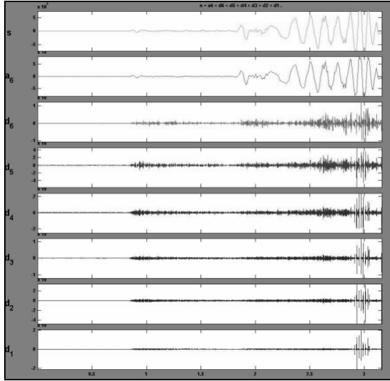
Şekil 13. 17.08.2000 tarihinde meydana gelen büyüklüğü M_w : 7.4 olan depremin doğu bileşen kaydına uygulanmış dalgacık dönüşümü çıktısı.
