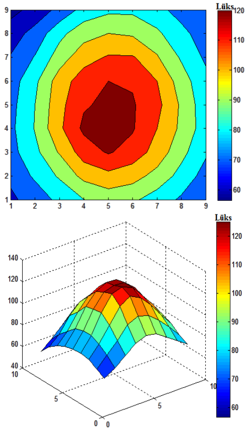
Şekil 6: Karma aydınlatılan krem rengi iç mekândaki aydınlık düzeyi dağılımlarının iki ve üç boyutlu grafikleri.
