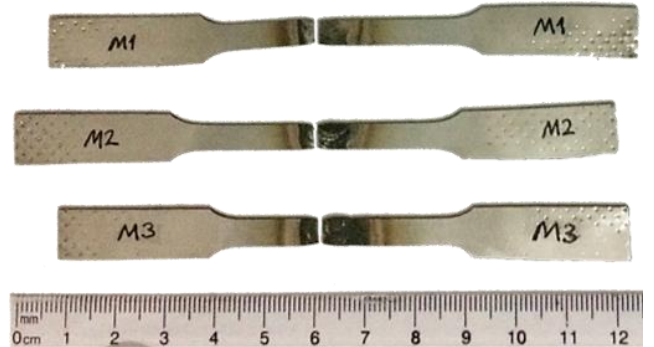
Şekil 9. Manuel Olarak Birleştirilen Numunelerin Çekme Testi Sonrası Görüntüleri
