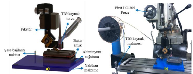
Şekil 1. Kaynaklı Birleştirme İşlemlerinde Kullanılan Portatif Fiktür a) Fiktür Tasarımı b) Frezeyle Bağlanmış Hali
