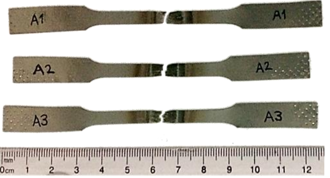
Şekil 8. Yarı-Otomatik Olarak Birleştirilen Numunelerin Çekme Testi Sonrası Görüntüleri
